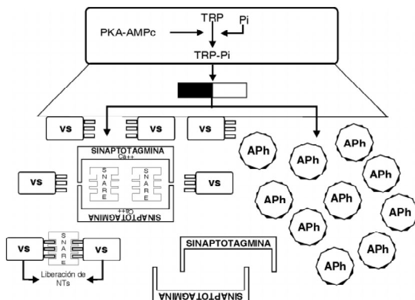
Figura 3. En el momento en que las TRPs-AMPC se unen al elemento regulador del AMPc dentro del núcleo, genes inductores codifican varias respuestas. Inicialmente el \text{Ca}^{++} se une a la sinaptotagmina evitando que las VS se fusionen entre sí, pero cuando el \text{Ca}^{++} es liberado de los SNARE, las \alpha -SNAP promueven la fusión de las VS permitiendo la liberación del NT. Finalmente, genes efectores sintetizan las enzimas necesarias para catabolizar a la \text{S}_r y liberar a la \text{S}_c , induciendo los procesos de autofosforilación de distintas PK, como la PKC-AMPC.
