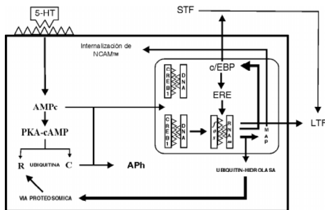
Figura 2. La PKA-AMPC además de fosforilar a los canales K s y K A activa a genes efectores capaces de iniciar un proceso de LTF en tres diferentes fases: 1. Iniciación, en la que la represión de la CREB2 permite la activación de la CREB1; 2. Consolidación, que se caracteriza porque genes de respuesta inmediata promueven la síntesis de la hidrolasa carboxiterminal de la ubiquitina que cataboliza a la R s y libera a la C s de la PKA-AMPC, induciendo su autofosforilación (APh); y 3. Estabilización, durante la cual la internalización de las NCAM TM permite la defasciculación y crecimiento de las arborizaciones dendríticas, mientras que con la posterior externalización de las mismas moléculas induce la conformación de nuevos contactos sinápticos.
