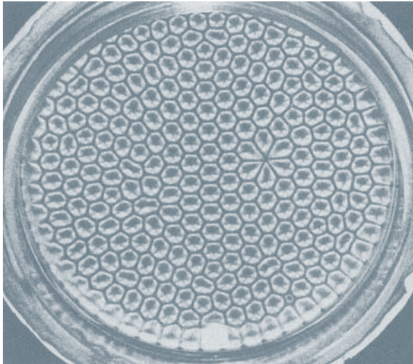
Figura 1.1. Celdas de convección de Rayleigh-Bénard de un fluido calentado desde abajo, contenido en una caja de Petri. Es notable la organización en forma de celdas hexagonales, como en un panal de abejas; un resultado similar se obtiene al enfriar el fluido desde la superficie. Se han empleado diminutas hojuelas de una densidad similar a la correspondiente al fluido, con el fin de visualizar las corrientes; existe una dependencia no trivial con las condiciones de frontera, es decir, con la forma del recipiente en la selección de estructura, el patrón de las celdas de convección.
